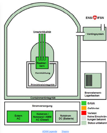
Darstellung 40: Liste der Systeme und Komponenten (links), deren Statusbeurteilung zur automatischen Einfärbung der Anlagengrafik (rechts) führt (Beispieldarstellung Druckwasserreaktor).
