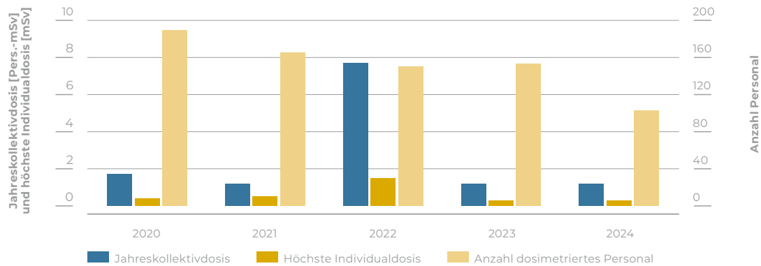
Anlagenbezogene Jahreskollektivdosis, Anzahl dosimetriertes Personal und höchste Individualdosis – Hotlabor
