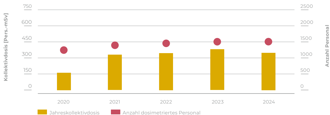
Darstellung 16: Jahreskollektivdosen und Anzahl dosimetriertes Personal im KKG in den letzten fünf Jahren.
