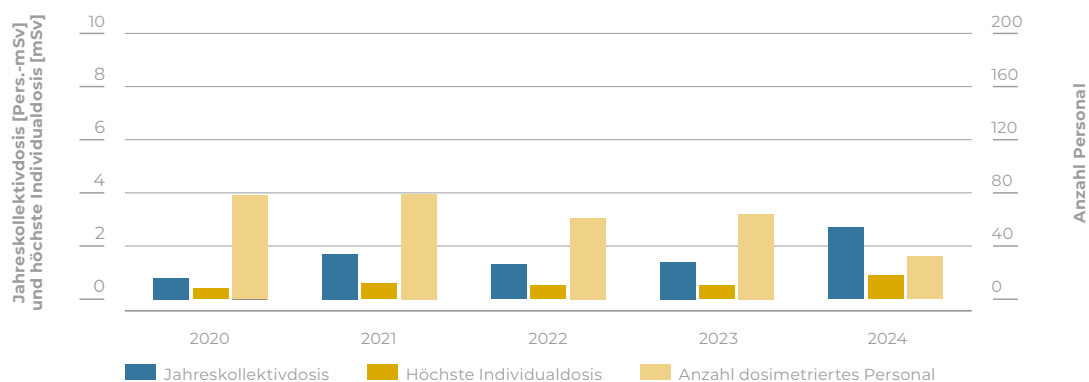
Anlagenbezogene Jahreskollektivdosis, Anzahl dosimetriertes Personal und höchste Individualdosis – AERA
