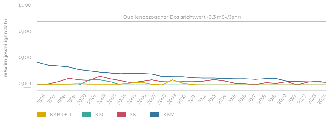
Darstellung 34: Berechnete Dosen für die meist- betroffenen Personen 1 in der Um- gebung der schweizeri- schen KKW.
