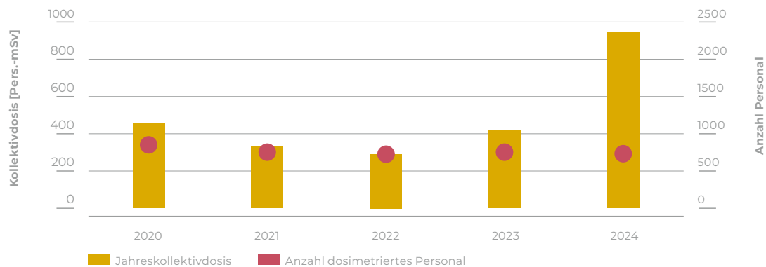
Darstellung 25: Summe der Kollektivdosen und Anzahl beruflich strahlenexponierter Personen im KKM in den letzten fünf Jahren.
