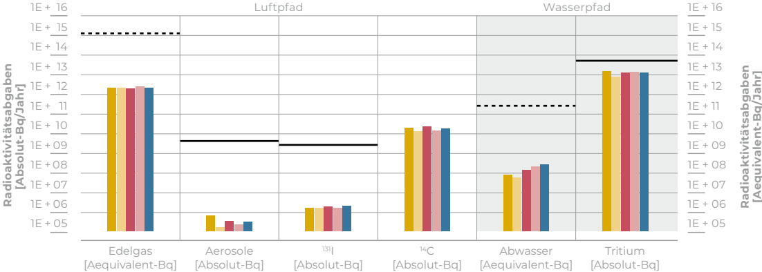
Darstellung A1: Abgaben der schwei- zerischen KKW an die Atmosphäre und über das Abwasser in den letzten fünf Jahren (2020 bis 2024) im Ver- gleich mit den Jahresabgabe- limiten.
