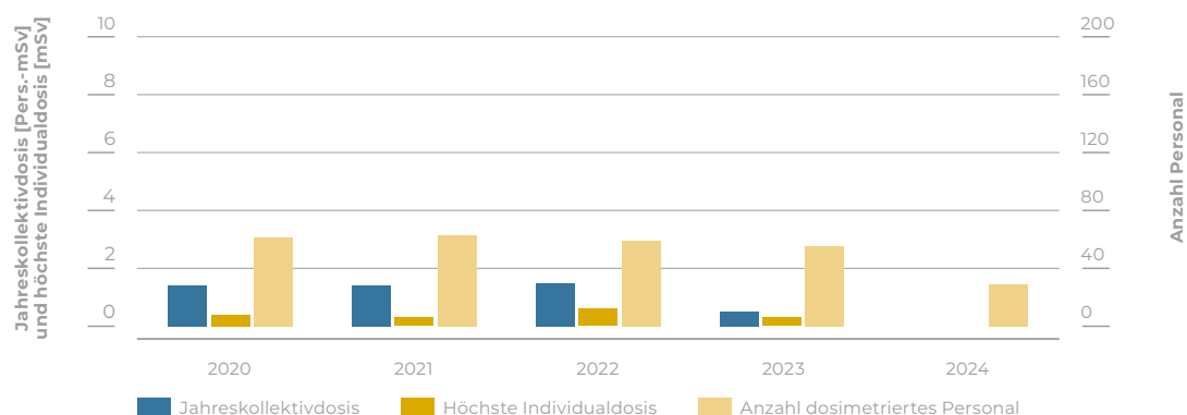
Anlagenbezogene Jahreskollektivdosis, Anzahl dosimetriertes Personal und höchste Individualdosis – VVA
