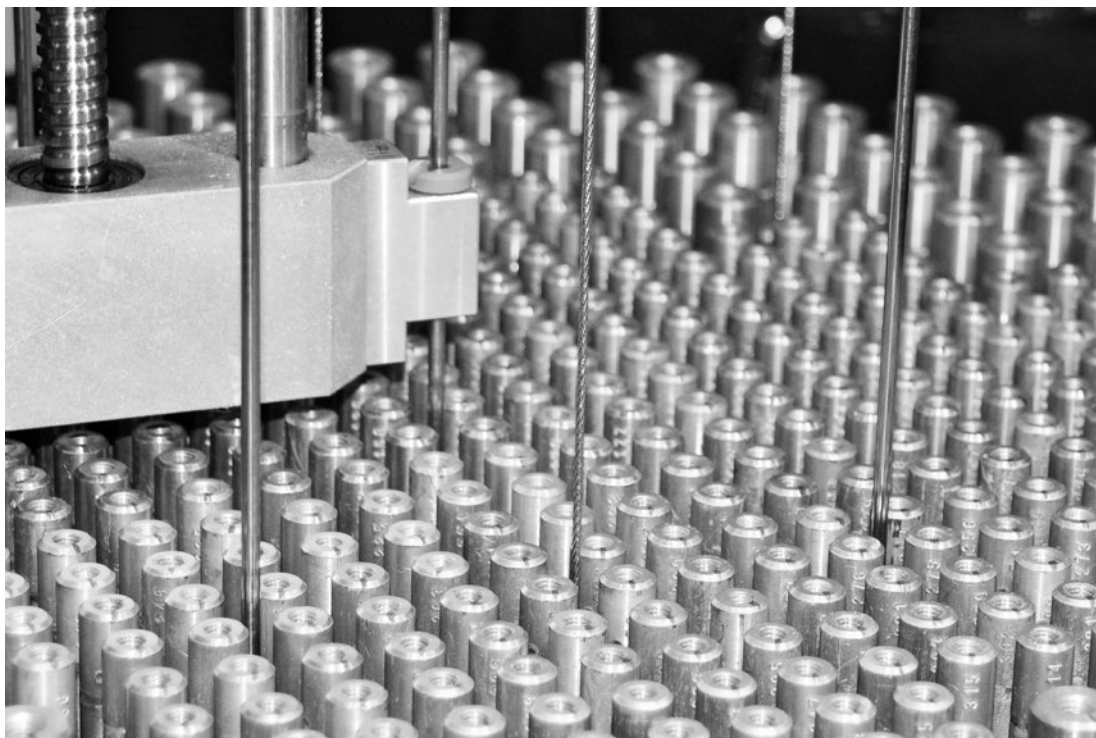
Bild 22: Nahaufnahme des Reaktorkerns des CROCUS mit dem TRAX-System (Translation RAdial aXial) zum Einfahren einer Spaltkammer in den Reaktor.
