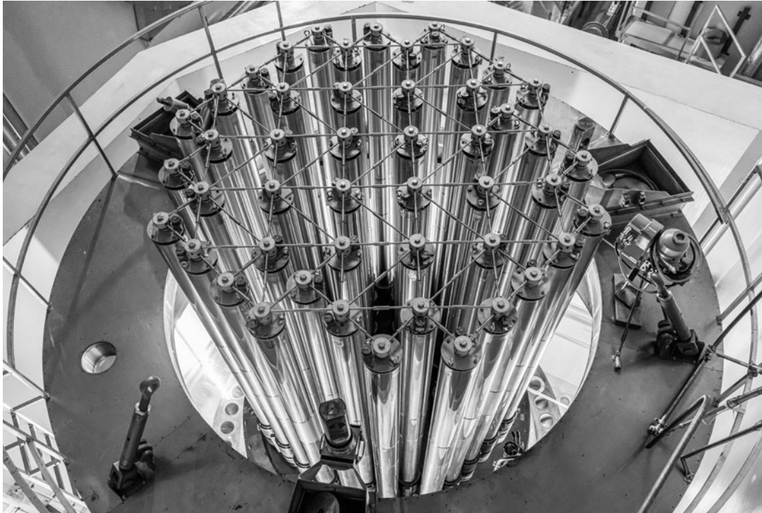
Bild 15: Reaktor- deckel am Abstellplatz. Gut sichtbar sind hier die Steuerstab- führungs- rohre.
