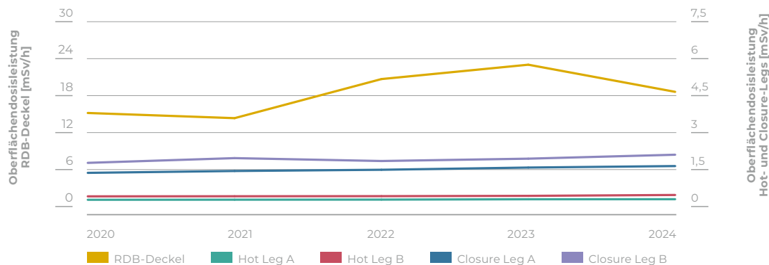
Darstellung 5: Verlauf der gemessenen Oberflächendosisleistung im KKB Block 2 am Reaktor-druckbehälter-Deckel (linke Achse) und an den Hauptkühlmittel-leitungen der Hot- und Closure-Legs (rechte Achse).
