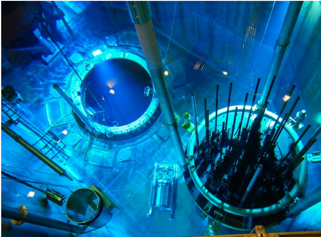
Bild 12: Geflutete Reaktorgrube mit offenem Reaktordruck- behälter im KKB Block 1.
