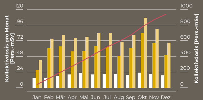
Kollektivdosis Eigen- und Fremdpersonal des KKM in 2024
