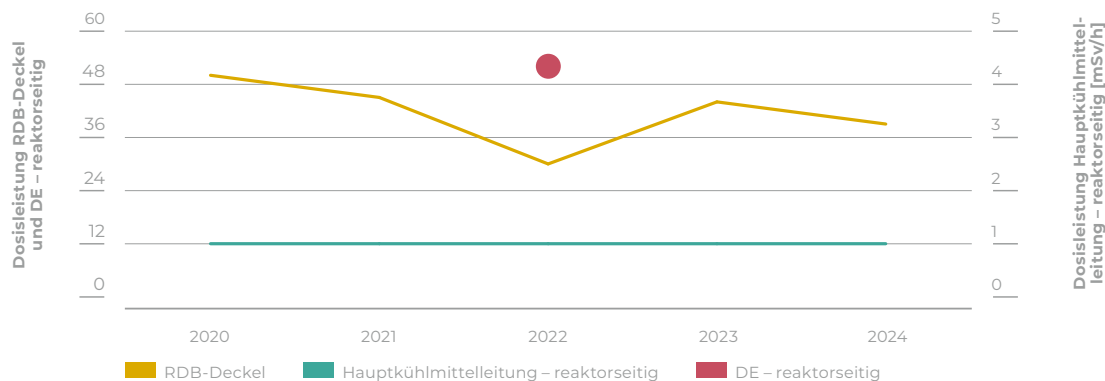
Oberflächendosisleistungen an Komponenten des Primärkreislaufs des KKG
