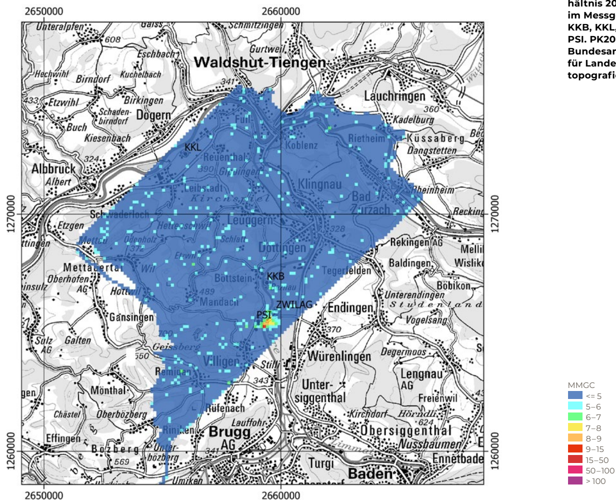
MMGC-Verhältnis im Messgebiet KKB, KKL, ZZL und PSI
