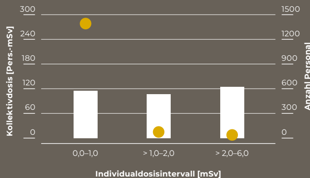
Kollektivdosen und Anzahl dosimetriertes Personal im KKG
