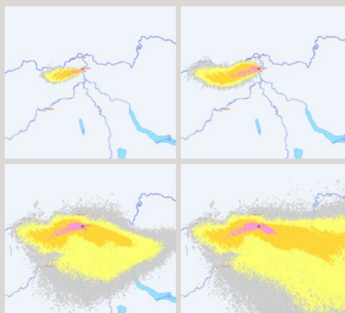
Darstellung 42: Beispiel einer JRODOS- Simulation für das KKB.
