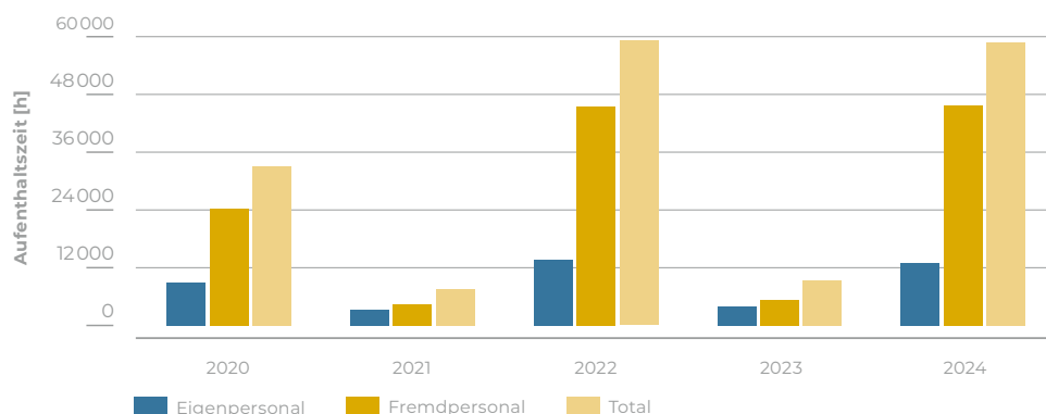
Aufenthaltszeit in der kontrollierten Zone während den geplanten Stillständen im KKB Block 1
