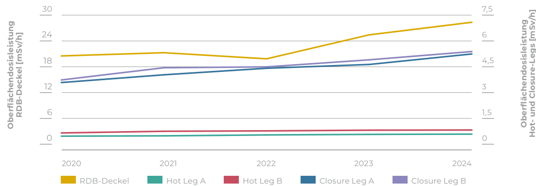
Darstellung 4: Verlauf der gemessenen Oberflächendosisleistung im KKB Block 1 am Reaktor-druckbehälter-Deckel (linke Achse) und an den Hauptkühlmittel-leitungen der Hot- und Closure-Legs (rechte Achse).
