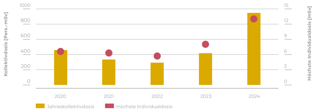
Darstellung 24: Jahreskollektiv- (Pers.-mSv) und höchste Individualdosen (mSv) im KKM in den letzten fünf Jahren.
